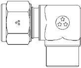
EQSWS - page 43 Coude à souder par emboîtement SW Socket Welding Elbow Winkel-Verschraubung SW
