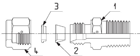
1 Corps 2 Bague avant 3 Bague arrière 4 Ecrou
